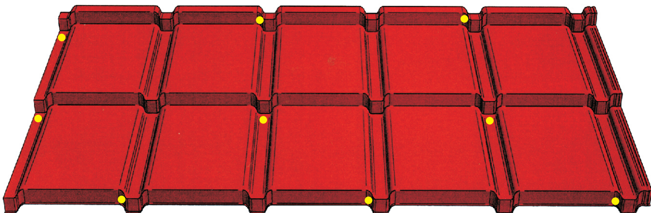
Rys. 5. Rozmieszczenie wkrętów
